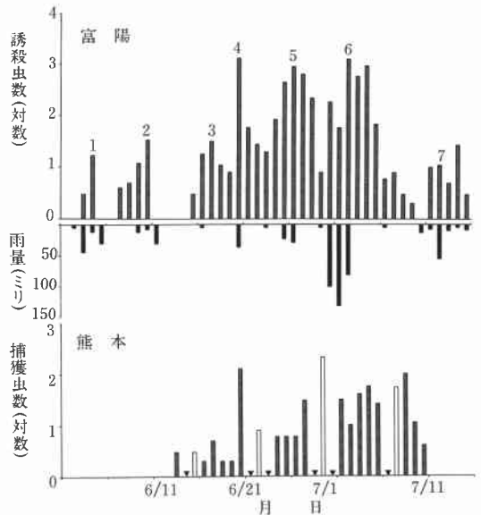
第1図 中国水稻研究所（富陽）における予察灯によるセジロウンカの日別誘殺虫数と雨量、および熊本県農業研究センター（熊本）におけるネットトラップによるセジロウンカの日別捕獲虫数。富陽のグラフ中の番号1～7は、飛来波を示す。熊本のグラフ中、白抜きの棒グラフは、▼印を付した前日を含む2日間、あるいは前後日を含む3日間の合計獲得虫数を示す。
